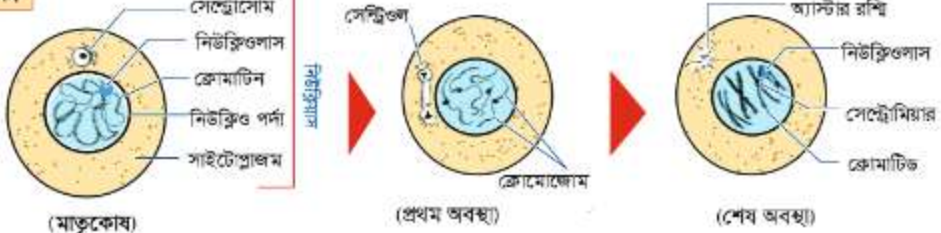
চিত্র 3.01-02: প্রোফেজ
