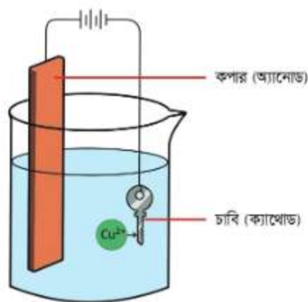
চিত্র 10.11: চাবির উপর কপার ধাতুর ইলেকট্রোপ্লেটিং।
