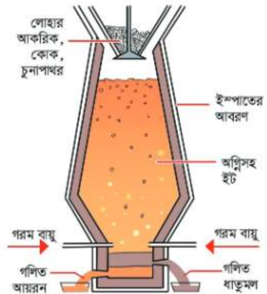
চিত্র 10.09: ব্যাত্যাচুপ্তিতে আয়রন নিষ্কাশন।
