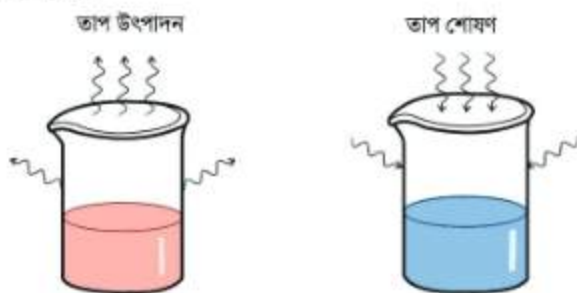
চিত্র 8.01: তাপ উৎপাদন ও তাপ শোষণ।
