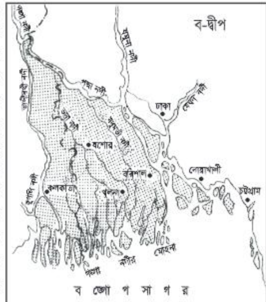
চিত্র ৪.১২ : ব-দ্বীপ
