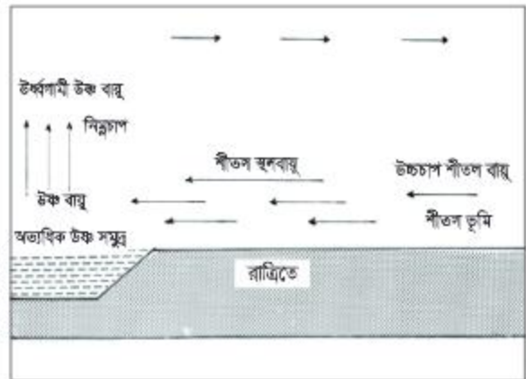
চিত্র ৫.৯ : স্থলবায়ু
