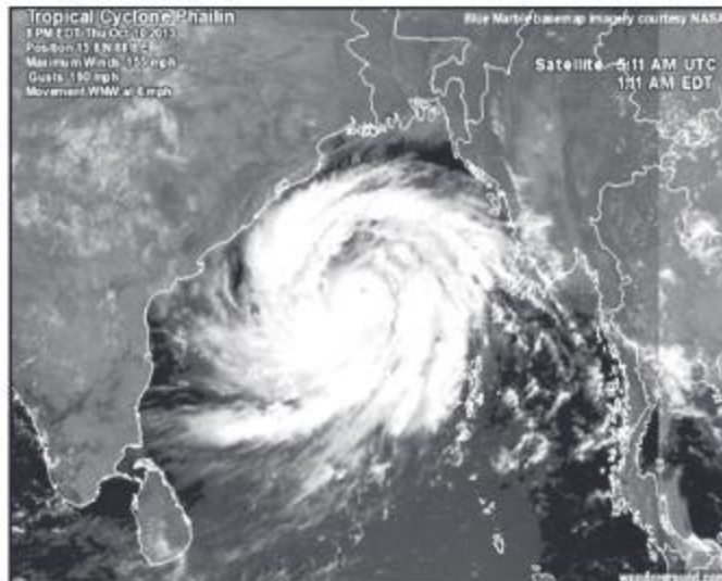
চিত্র ১৪.১ : ঘূর্ণিঝড়
