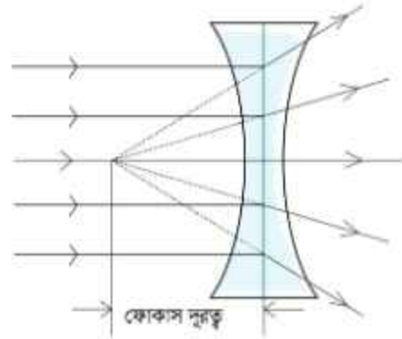
চিত্র 9.18: অবতল লেন্সের ভেতর দিয়ে হওয়ার সময় সমান্তরাল রশ্মি ছড়িয়ে পড়ে।
