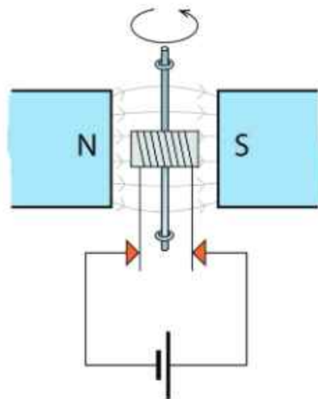
চিত্র 12.11: একটি বৈদ্যুতিক মোটর।
