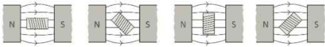
চিত্র 12.10: বৈদ্যুতিক মোটর একটি তাড়িতচুম্বকের ভেতর দিয়ে এমনভাবে পরিবর্তী বিদ্যুৎ প্রবাহ করানো হয়, যেন সব সময়েই এটি ঘুরতে থাকে।
