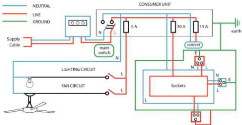
চিত্র 11.17: একটি বাসায় বিদ্যুৎ সরবরাহ করার জন্য সম্ভাব্য বিদ্যুৎ বতনী।
