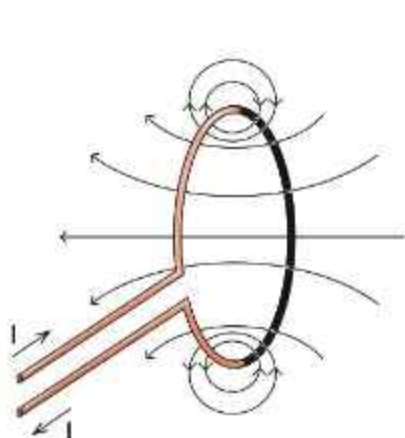
চিত্র 12.05: লুপের ভেতর দিয়ে বিদ্যুৎপ্রবাহের কারণে তৈরি চৌম্বক ক্ষেত্র।
